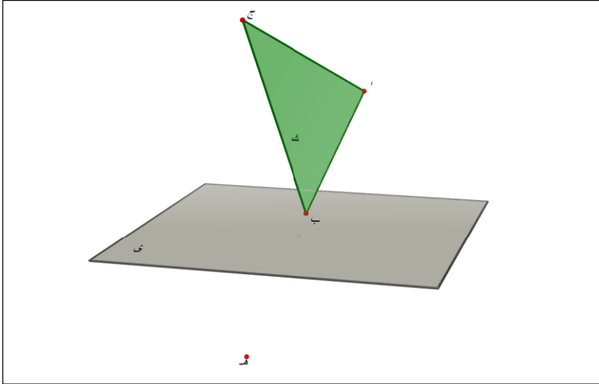
شكل (٢) : مستويان يشتركان في نقطة
