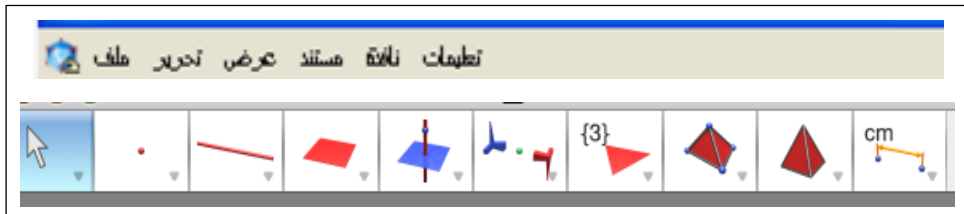
شكل ( ١ ): صندوق الأدوات لواجهة برنامج CABRI 3D
