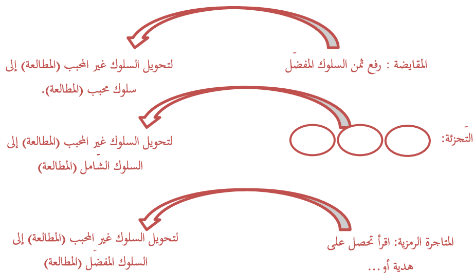
شكل ١: تعديل السلوك
