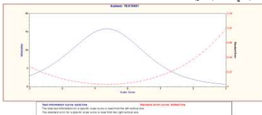
شكل (1) دالة المعلومات والخطأ المعياري للاختبار القدرة العقلية
