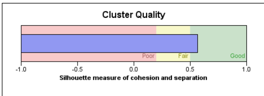
شكل (٢): جودة القطاعات الناتجة بمخرج تحليل التجمعات.
