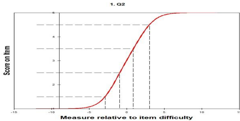
شكل (2): منحنى خصائص المفردة (2) في المقياس وفقاً لنموذج مقياس التقدير
