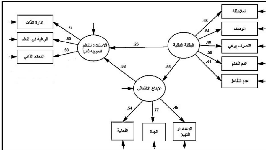
شكل (٢): القيم المعيارية للتأثيرات المباشرة لمتغيرات الدراسة
