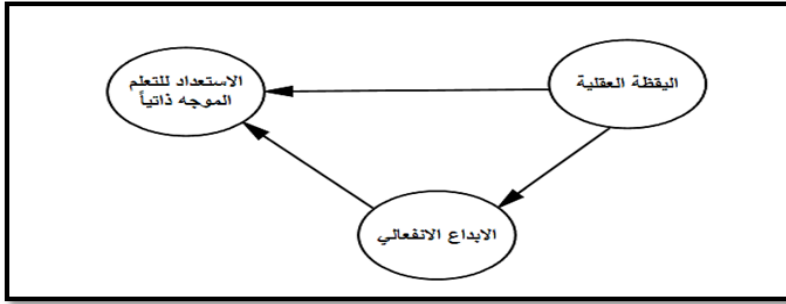
شكل (١): النموذج البنائي للعلاقة بين متغيرات الدراسة
