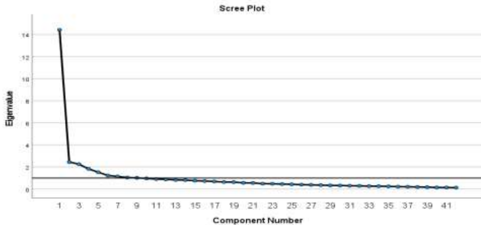
شكل (٣) (Scree plot) للتحليل العاملي الاستكشافي لمقياس التلكؤ الأكاديمي
