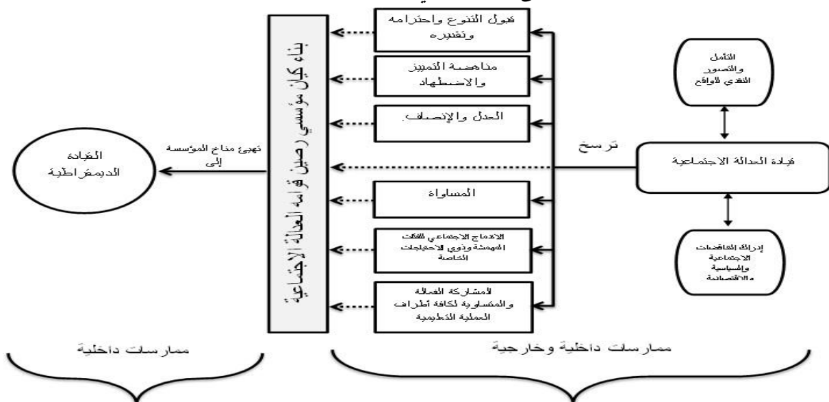
شكل (٢) يوضح العلاقة التفاعلية بين قيادة العدالة الاجتماعية والقيادة الديمقراطية.
